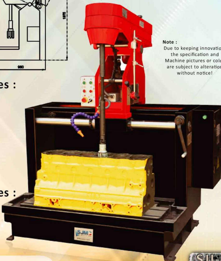
HR70D ( \Phi 66 - \Phi 140 mm)
